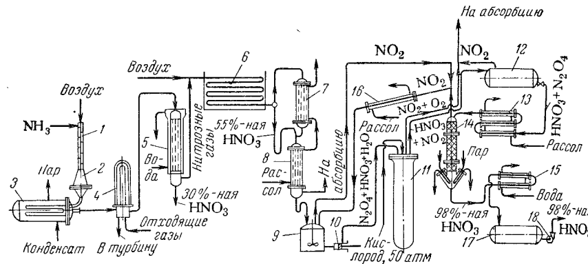
Рис. VIII-36. Схема производства концентрированной азотной кислоты из нитрозных газов, полученных под давлением:
