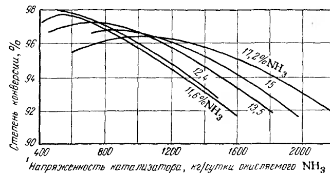
Рис. II-10. Зависимость степени конверсии аммиака от напряженности катализатора и содержания аммиака в газовой смеси при 900^\circ \text{C} .
