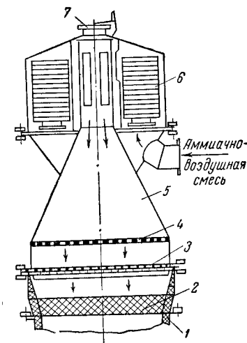
Рис. VI-2. Контактный аппарат (диаметр 2,8 м):
