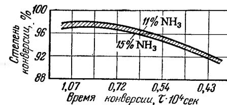
Рис. II-9. Зависимость степени конверсии аммиака от времени конверсии при постоянном отношении \text{O}_2 : \text{NH}_3 = 2 и при 900° С.
