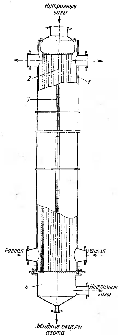
Рис. VIII-29. Конденсатор окислов азота: 1 — кожух; 2 — трубы; 3 — линия разъема кожуха; 4 — отделитель жидкости.
