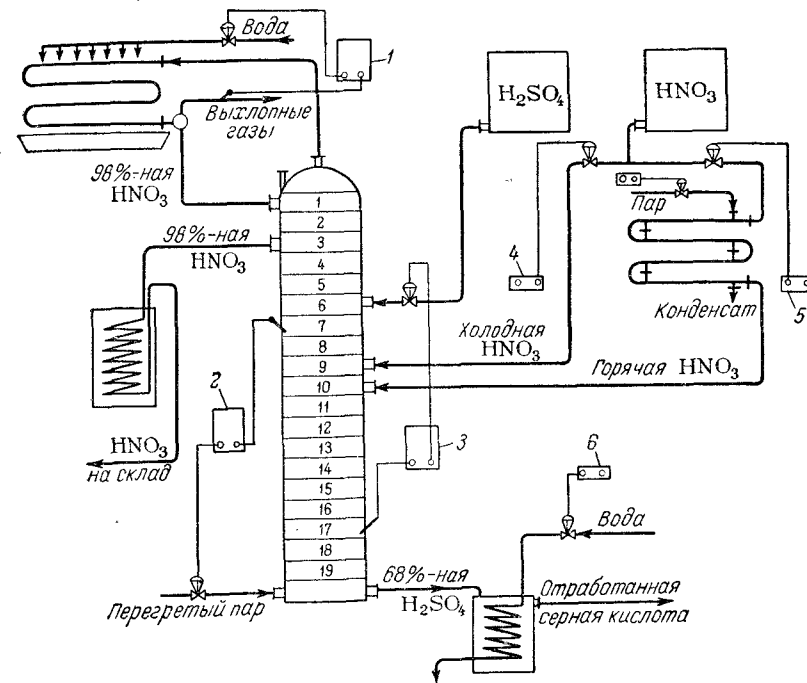
Рис. VII-11. Схема автоматического управления агрегатом концентрирования разбавленной азотной кислоты:
