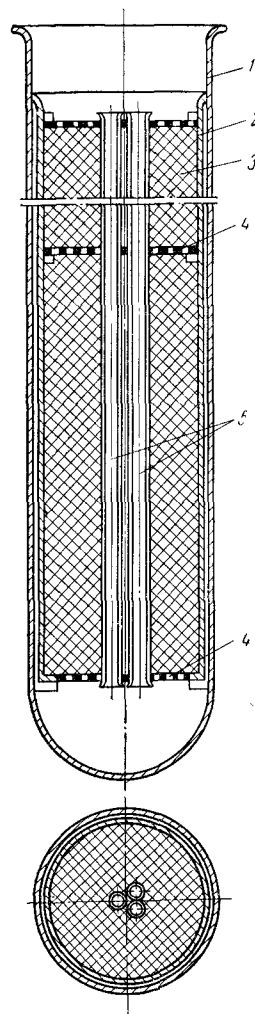
Рис. VIII-20. Автоклав пленочного типа:
