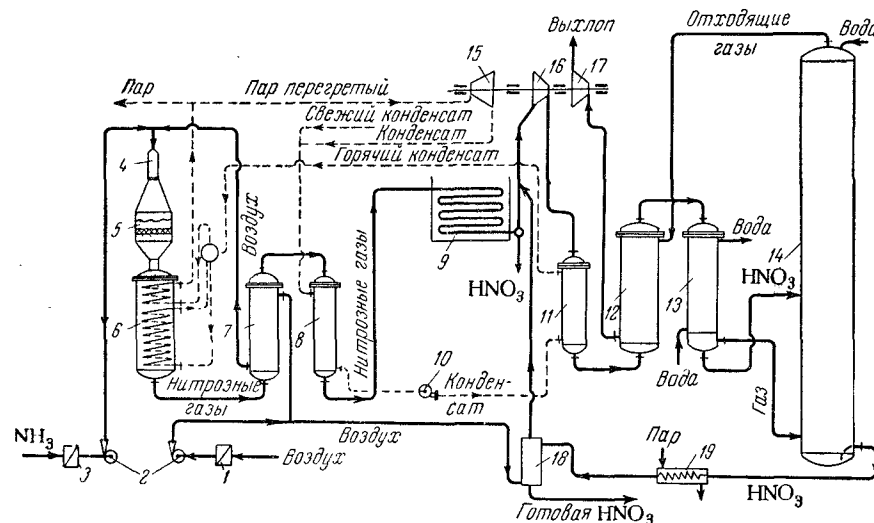
Рис. VI-19. Схема получения азотной кислоты по методу Кюльмана: 1—фильтр для воздуха; 2—воздушный и аммиачный вентиляторы; 3—фильтр аммиака; 4—смеситель; 5—конвертор; 6—паровой котел; 7—воздушный теплообменник; 8—первый подогреватель конденсата; 9—холодильник-конденсатор; 10—насос для питания котла-утилизатора; 11—теплообменник конденсата; 12—теплообменник отходящих газов; 13—плоченый холодильник-окислитель; 14—абсорбционная колонна; 15—паровая турбина; 16—нитрозный турбокомпрессор; 17—турбина рас циркуля; 18—продуктовая колонна; 19—подогреватель кислоты.
