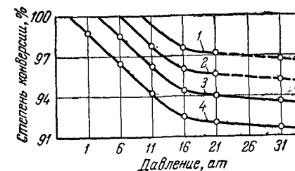
Рис. 11-13. Зависимость степени конверсии NH 3 от давления и температуры при оптимальном времени катализа: 1 — при 1010° С; 2 — при 980° С; 3 — при 950° С; 4 — при 900° С.
