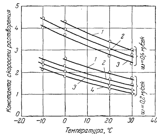
Рис. IV-14. Зависимость константы скорости растворения NO_2 от температуры, концентрации кислоты и линейной скорости газа W :
