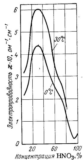
Рис. IV-25. Электропроводность водных растворов азотной кислоты (по данным О. П. Чану-квадзе).
