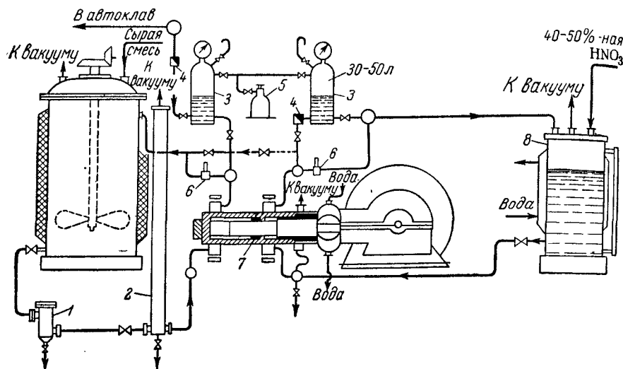
Рис. VIII-26. Схема подачи раствора двухкамерным насосом системы И. П. Сидорова в автоклав непрерывного действия:
