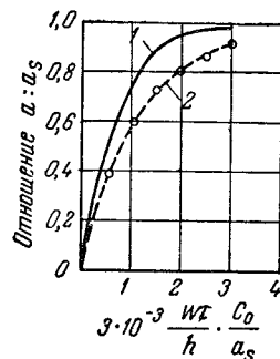
Рис. V-5. Поглощение NO 2 адсорбентом:
