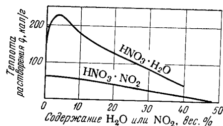
Рис. IV-29. Дифференциальная теплота растворения ( q в кал/г \text{NO}_2 или \text{H}_2\text{O} ) жидкой \text{NO}_2 в системе \text{HNO}_3\text{--NO}_2 и воды в системе \text{HNO}_3\text{--H}_2\text{O} .
