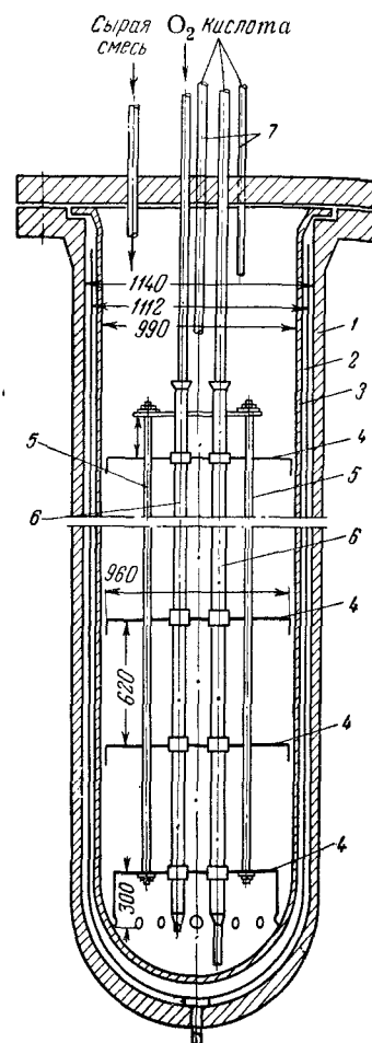
Рис. VIII-35. Автоклав непрерывного действия с ситчатыми тарелками: 1 — корпус; 2 — защитный стакан; 3 — реакционный стакан; 4 — ситчатые тарелки; 5 — распорные штанги; 6 — чехольные трубы (каналы); 7 — переливные трубы.
