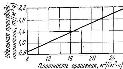
Рис. VIII-21. Зависимость удельной производительности автоклава с орошаемой поверхностью от плотности орошения (концентрация продукции 98—99%, соотношение N_2O_4:H_2O = 7,8-8,9 , давление 40 ат).
