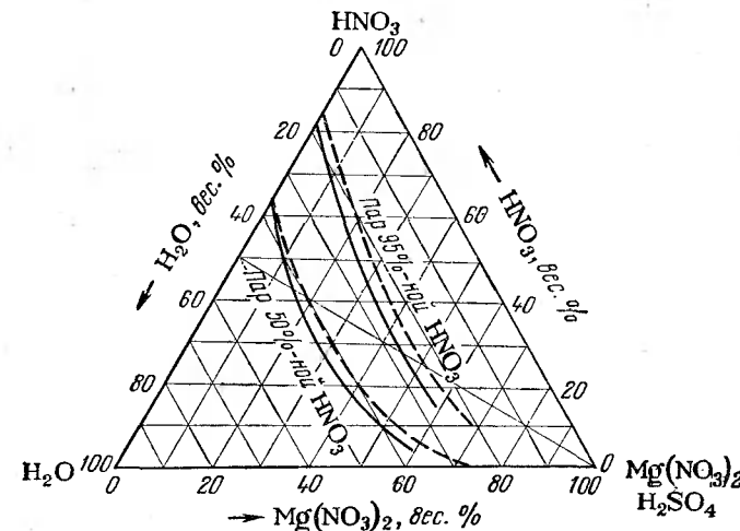
Рис. VII-15. Равновесная концентрация паров азотной кислоты над тройной смесью \text{HNO}_3\text{—H}_2\text{O—Mg}(\text{NO}_3)_2 (пунктирные линии относятся к смеси \text{HNO}_3\text{—H}_2\text{O—H}_2\text{SO}_4 ).
