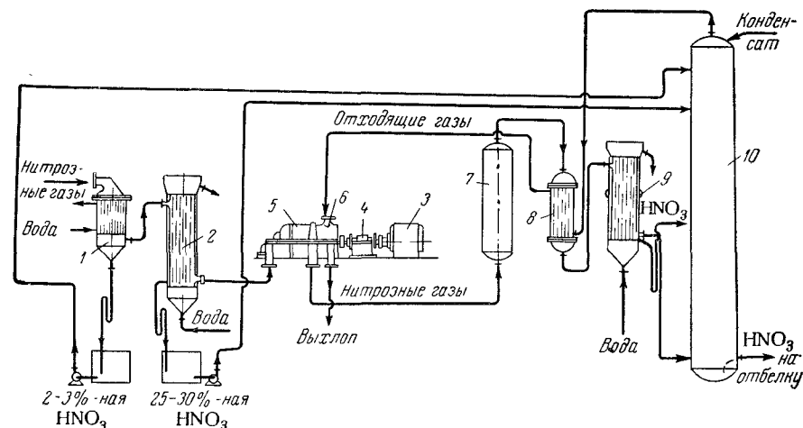
Рис. VI-17. Схема установки для получения разбавленной азотной кислоты комбинированным способом:
