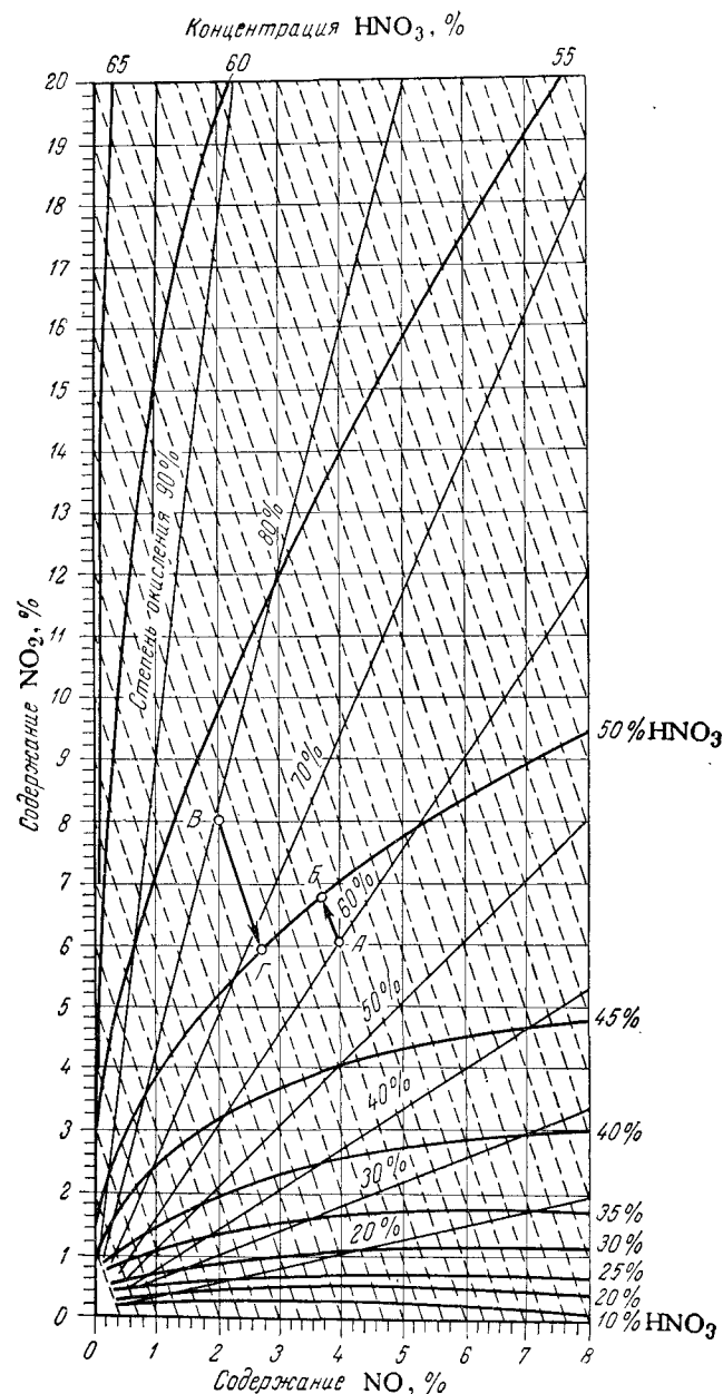
Рис. IV-5. Номограмма для определения соотношения окиси и двуокиси азота над раствором азотной кислоты в условиях равновесия при 25° С (пунктиром показаны линии изменения состава газа при переходе его в равновесное состояние с кислотой).
