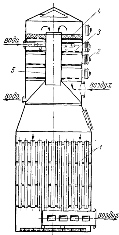
Рис. II-14. Комбинированный аппарат для очистки воздуха: 1 — матерчатый фильтр; 2 — лаз; 3 — ситчатая тарелка; 4 — керамические кольца; 5 — труба для воздуха.
