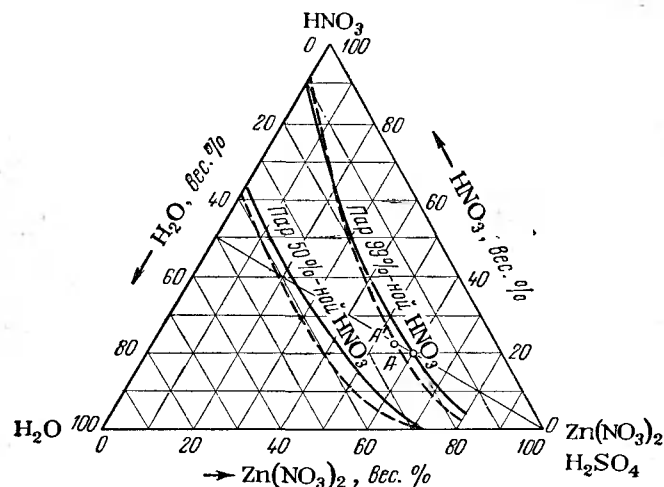
Рис. VII-14. Равновесная концентрация паров азотной кислоты над тройной смесью \text{HNO}_3\text{—H}_2\text{O—Zn}(\text{NO}_3)_2 (пунктирные линии относятся к смеси \text{HNO}_3\text{—H}_2\text{O—H}_2\text{SO}_4 ).
