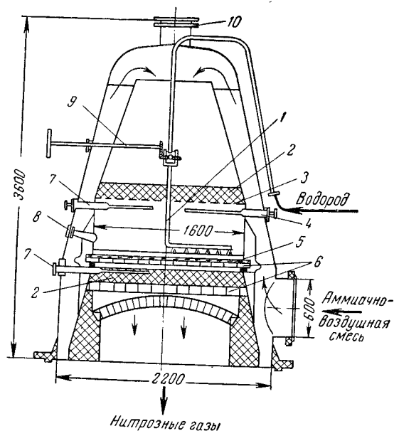
Рис. VI-10. Конвертор:
