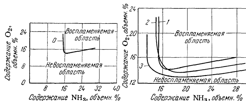
Рис. II-8. Области воспламенения аммиачно-воздушной смеси: 1 — температура смеси 23,8° С, давление 2 ат; 2 — t = 23,8^{\circ} С, P = 8 ат; 3 — t = 160^{\circ} С, P = 8 ат; 0 — t = 23,8^{\circ} С, P = 1,05 кгс/см 2 .
