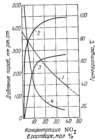
Рис. VIII-8. Парциальные давления паров окислов азота и азотной кислоты над растворами \text{NO}_2 в азотной кислоте при температуре кипения: 1 — температура кипения; 2 — давление паров \text{NO}_2 ; 3 — давление паров \text{N}_2\text{O}_4 ; 4 — давление паров \text{HNO}_3 .
