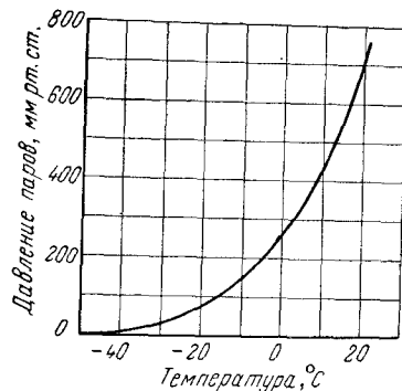
Рис. III-9. Давление паров над жидкой четырехокисью азота.
