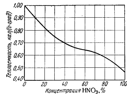
Рис. IV-24. Теплоемкость водных растворов азотной кислоты.
