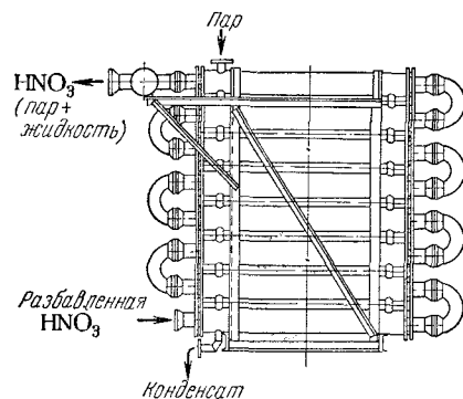
Рис. VII-7. Испаритель разбавленной азотной кислоты.
