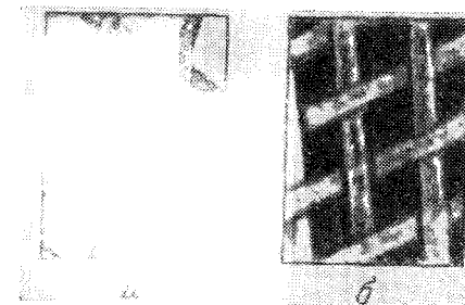
Рис. II-4. Вид платиновой сетки в увеличенном виде: а — неактивированная сетка; б — активированная сетка.
