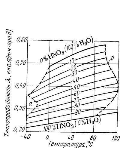
Рис. IV-27. Теплопроводность водных растворов азотной кислоты: а — кривая точек замерзания; б — кривая точек кипения.
