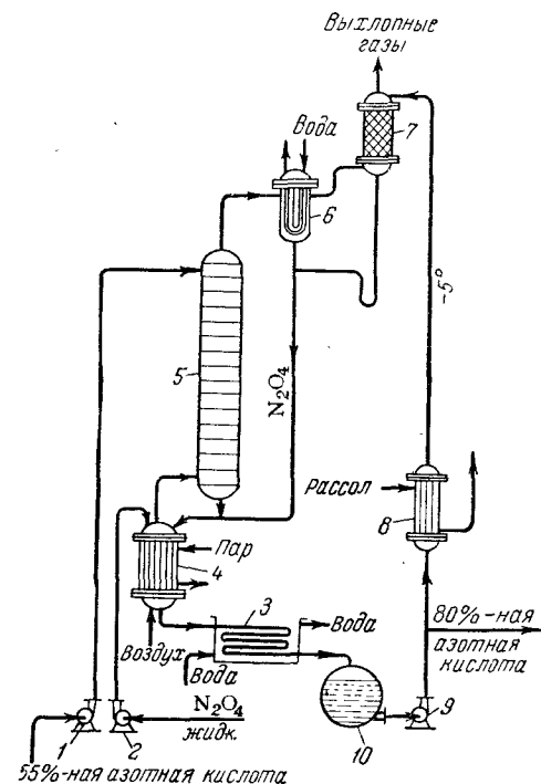
Рис. VII-12. Схема получения 80%-ной азотной кислоты из 55%-ной:
