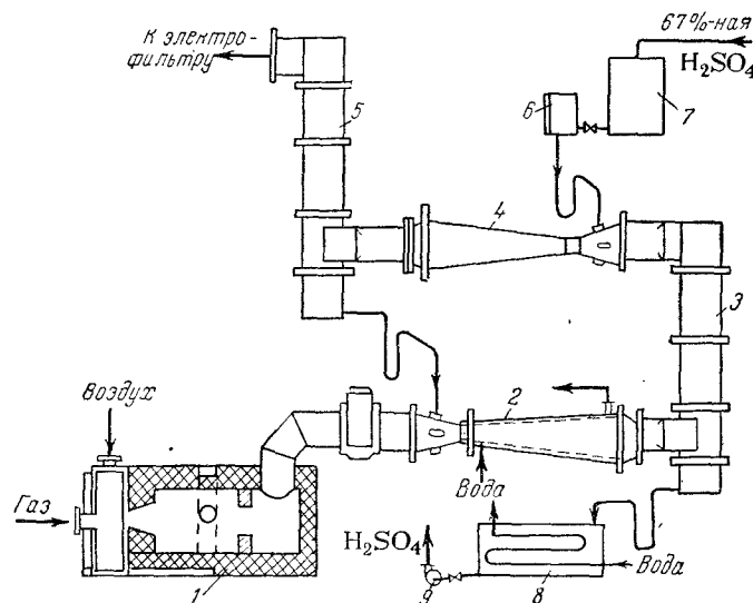
Рис. VII-23. Схема процесса капельного концентрирования серной кислоты в трубках Вентури:
