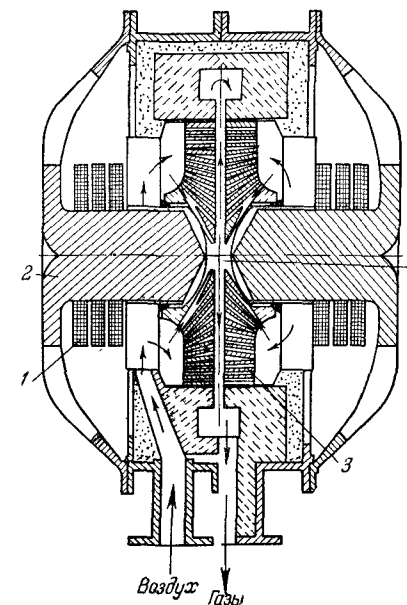
Рис. I-3. Печь Х. Биркелянда и С. Эйде для синтеза окиси азота: 1 — электрообмотка; 2 — полюсы; 3 — распределительная насадка; 4 — электрическая дуга.
