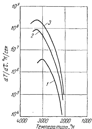
Рис. 1-8. Оптимальные режимы закалки окиси азота: 1 — 3000° К и 1 ат; 2 — 3300° К и 10 ат; 3 — 3300° К и 50 ат.
