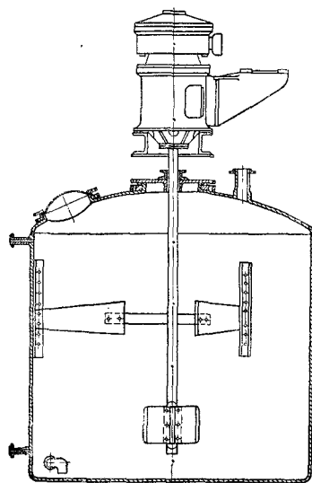
Рис. VIII-32. Смеситель.
