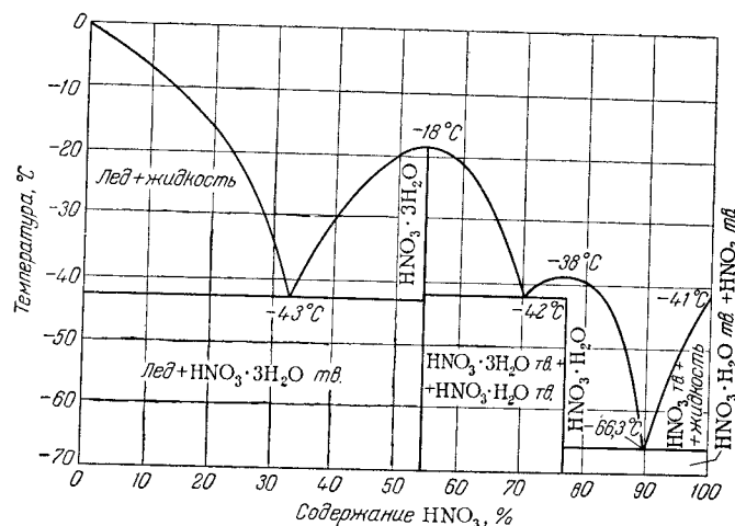
Рис. IV-17. Диаграмма кристаллизации системы \text{HNO}_3\text{--H}_2\text{O} .
