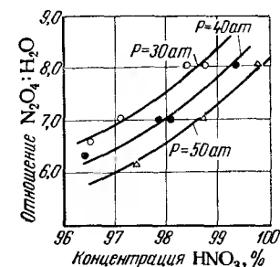
Рис. VIII-18. Зависимость концентрации автоклавной кислоты от соотношения \text{N}_2\text{O}_4 : \text{H}_2\text{O} и давления в автоклаве с затопленной насадкой (температура 70° C, число тарелок 11).
