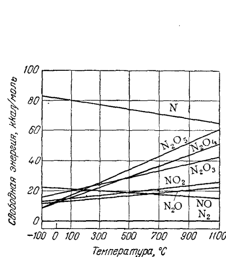
Рис. III-1. Термодинамическая устойчивость окислов азота.
