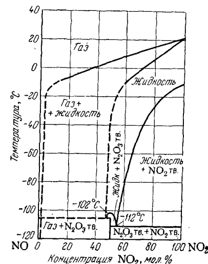
Рис. III-2. Диаграмма состояния системы NO—NO 2 при 1 атм.
