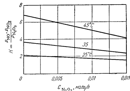
Рис. III-12. Зависимость константы равновесия реакции образования трехокси азота от температуры и концентрации N_2O_3 .
