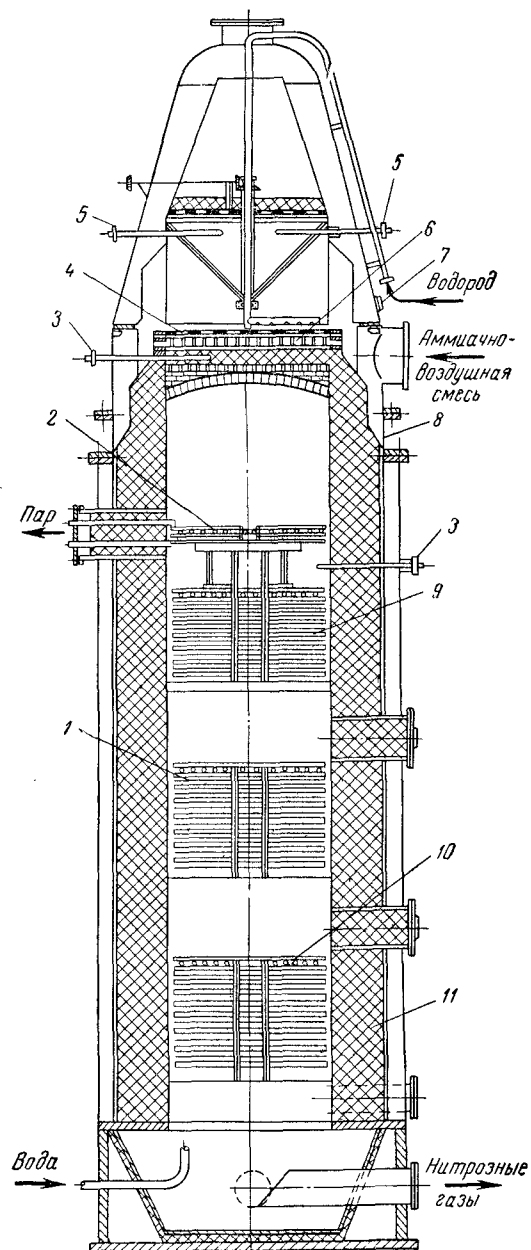
Рис. II-17. Контактный аппарат для окисления аммиака под давлением:
