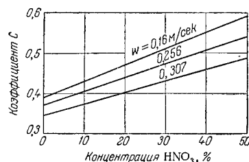
Рис. IV-8. Значения коэффициентов C для расчета абсорбционных колонн с тарелчатыми тарелками, работающих при 3,5 ат и 35—37° С.
