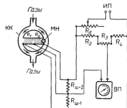
Рис. X-1. Схема газоанализатора типа МГК-2М:
