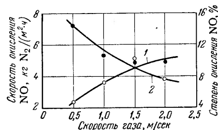
Рис. IV-2. Влияние линейной скорости газа в аппарате на степень и скорость окисления окиси азота в жидкой фазе при концентрации азотной кислоты 20%, температуре 30°С, парциальном давлении окислов азота 0,05 ат:
