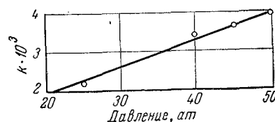
Рис. VIII-22. Зависимость константы скорости реакции от давления (температура 90°С, отношение N_2O_4:H_2O = 8 \div 8,5 ).
