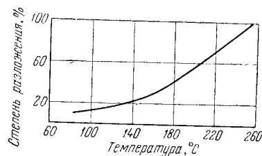
Рис. IV-30. Равновесная степень разложения азотной кислоты при различной температуре по реакции 2\text{HNO}_3 = \text{N}_2\text{O}_3 + \text{O}_2 + \text{H}_2\text{O} .
