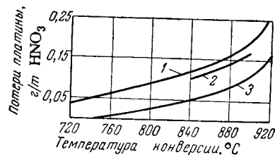
Рис. II-15. Зависимость потерь платины новых контактных сеток от температуры (диаметр нитей сеток 0,075 мм, число плетений 1024 на 1 см 2 ):
