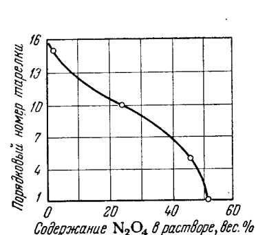
Рис. VIII-6. Содержание \text{N}_2\text{O}_4 в жидкости по высоте абсорбера.
