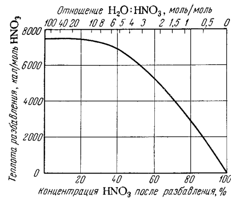
Рис. IV-23. Теплота разбавления азотной кислоты водой.
