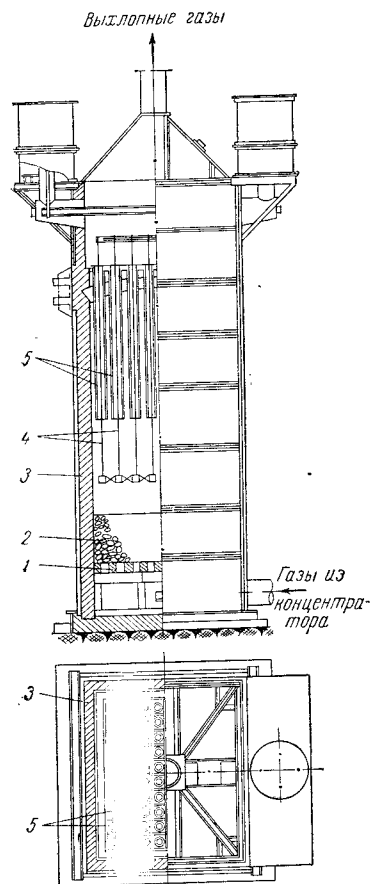
Рис. VII-21. Электрофильтр: 1 — колониковая решетка; 2 — кварц; 3 — андезитовая кладка; 4 — коронирующие электроды; 5 — осадительные электроды.
