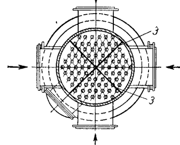
Рис. VI-4. Подогреватель воздуха: 1 — компенсатор; 2 — корпус; 3 — перегородки; 4 — трубки.
