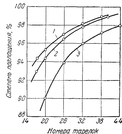
Рис. IV-37. Зависимость степени абсорбции окислов азота от числа ситчатых тарелок в колонне (температура 37^{\circ}\text{C} , высота перелива 35 мм, концентрация кислоты 50%) при различных линейной скорости газа и давлении:
