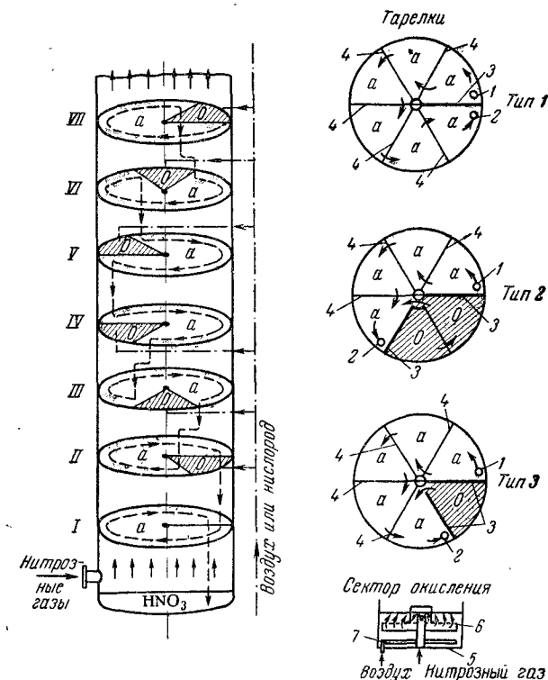
Рис. VI-20. Схема устройства абсорбционной колонны и отдельных тарелок: 0 — сектор окисления (заштрихован); а — сектор абсорбции; 1 — отверстие для приема кислоты с вышележащей тарелки; 2 — переток кислоты на нижележащую тарелку; 3 — высокие глухие перегородки; 4 — высокие перегородки с перетоками для кислоты (переток указан стрелками); 5 — глухая тарелка; 6 — ситчатая тарелка; 7 — труба для подвода воздуха или кислорода; I, II, III, ..., VII — тарелки по высоте колонны.
