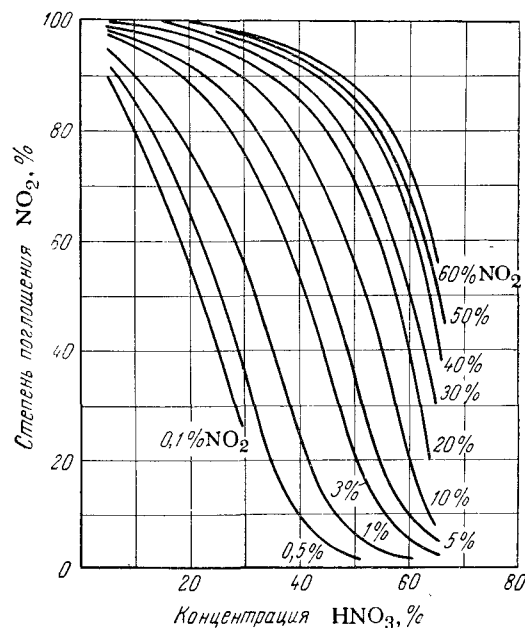
Рис. IV-6. Зависимость степени поглощения двуокиси азота от концентрации азотной кислоты в условиях равновесия при 35^\circ\text{C} и общем давлении газа 1 атм.
