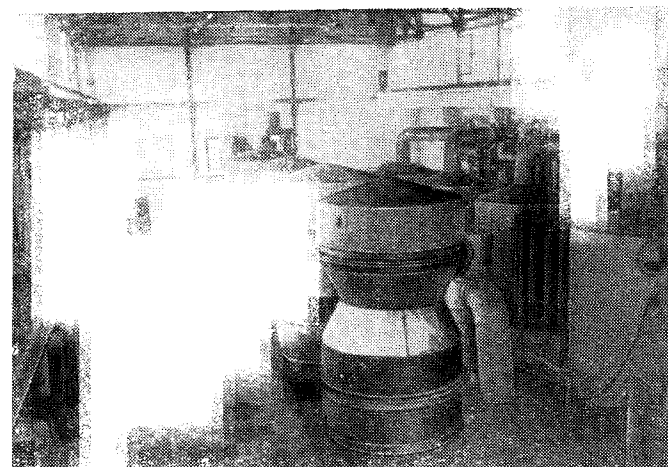
Рис. II-6. Общий вид контактного отделения, работающего при атмосферном давлении.
