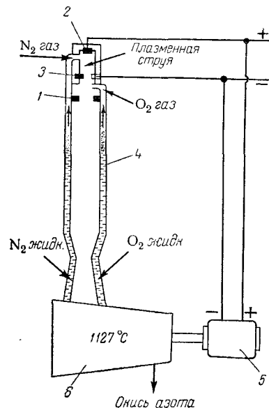
Рис. 1-6. Схема плазменного реактора для синтеза окиси азота: 1 — турбулизирующее кольцо; 2 — анод; 3 — катод; 4 — реактор; 5 — генератор постоянного тока; 6 — газовая турбина.
