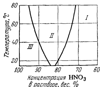
Рис. VIII-10. Изменение концентрации азотной кислоты в смеси N_2O_4 + H_2O + HNO_3 при протекании промежуточных реакций в процессе образования HNO_3 :
