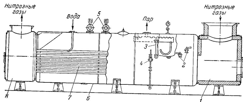
Рис. VI-3. Котел-утилизатор:
