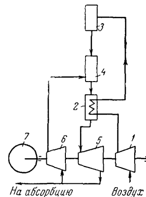
Рис. 1-10. Схема установки синтеза окиси азота в плазмотроне с закалкой холодными нитрозными газами: 1 — компрессор воздуха; 2 — теплообменник; 3 — плазмотрон; 4 — смеситель горячих и холодных нитрозных газов; 5 — газовая турбина; 6 — циркуляционный компрессор; 7 — электромотор.
