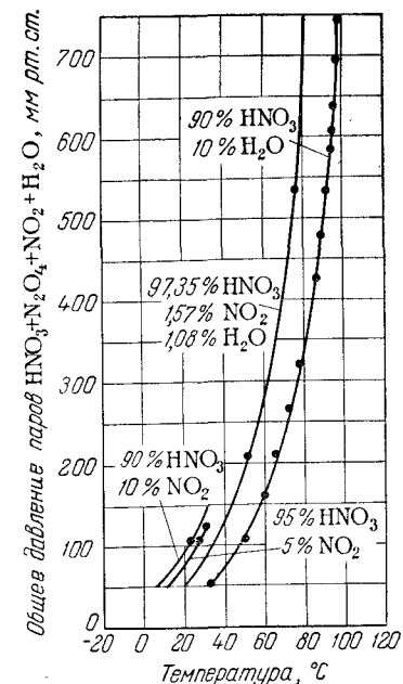
Рис. VIII-4. Общее давление паров над растворами HNO_3 + NO_2 + H_2O .
