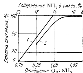
Рис. II-7. Зависимость степени окисления аммиака в окись азота от отношения O_2 : NH_3 в аммиачно-воздушной смеси при 900° С:
