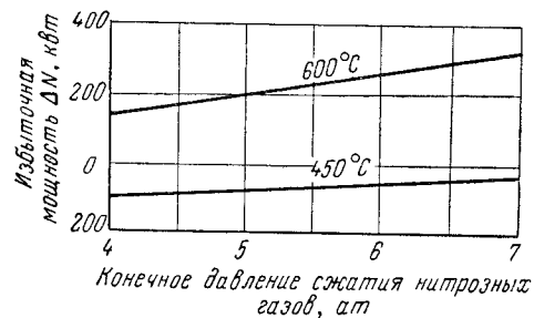
Рис. IV-38. Избыточная мощность на валу газовой турбины в зависимости от давления нитрозных газов в системе: 1 — при температуре газа на входе в газовую турбину 600° С; 2 — то же, при 450° С.
