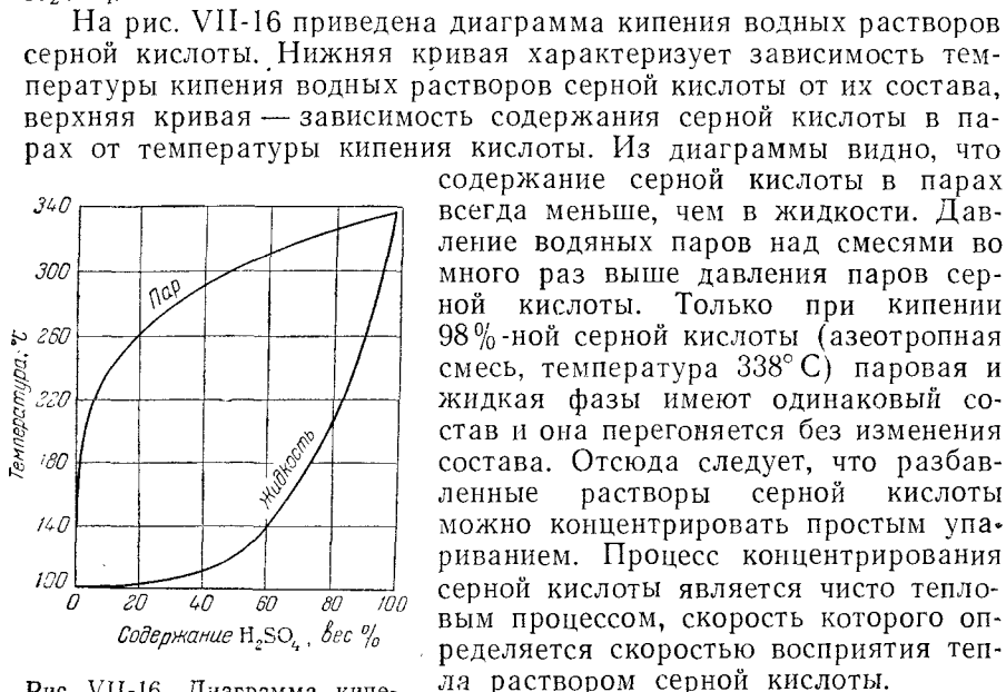
Рис. VII-16. Диаграмма кипения водных растворов серной кислоты.
