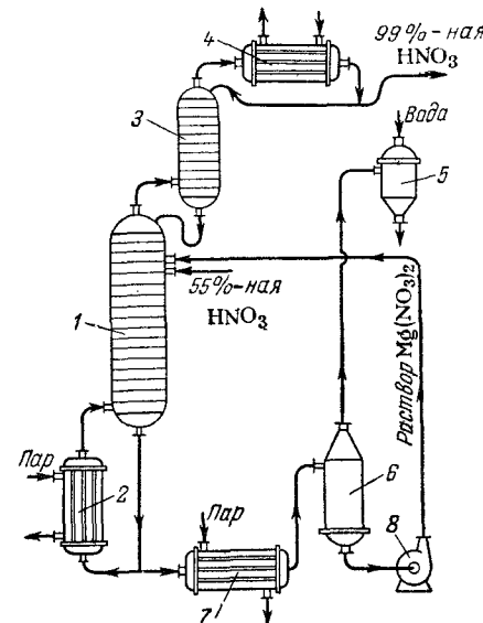
Рис. VII-13. Принципиальная схема получения концентрированной азотной кислоты при помощи нитрата магния:
