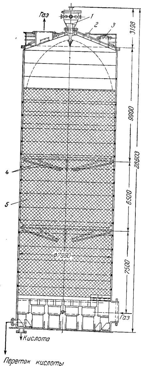
Рис. VI-6. Абсорбционная колонна:
