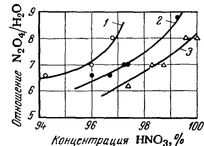
Рис. VIII-19. Влияние типа затопленной насадки автоклава на процесс кислотообразования (давление процесса 50 ат, температура 70° C): 1 — насадка из колец Рашига + 4 тарелки; 2 — насадка из 6 тарелок; 3 — насадка из 11 тарелок.
