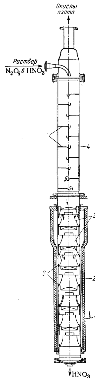
Рис. VIII-31. Отбелочная колонна: 1 — стальная рубашка; 2 — нагревательная часть с тарелками; 3 — тарелки; 4 — теплообменная часть с каскадными тарелками; 5 — каскадные полутарелки; 6 — уплотнения.
