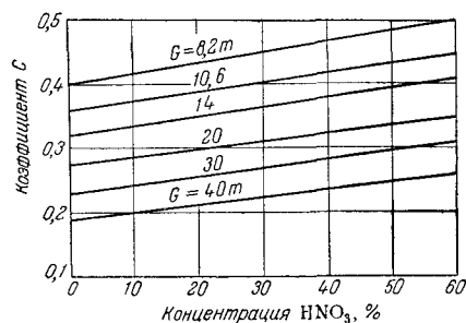
Рис. IV-7. Значение коэффициентов C для расчета абсорбционных колонн с барботажными колпачками, работающих при 7 ат и 30° С ( G — суточная производительность колонн, т моногидрата).
