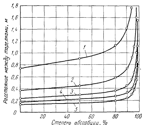
Рис. IV-13. Оптимальное расстояние между ситчатыми тарелками в абсорбционной колонне при поглощении окислов азота в зависимости от желаемой степени абсорбции на тарелке:
