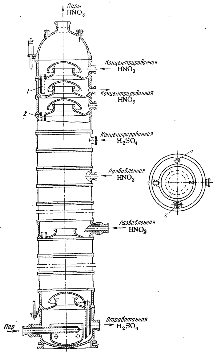
Рис. VII-9. Колонна барботажного типа для концентрирования азотной кислоты: 1, 2 — переточные трубки.
