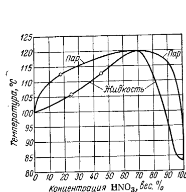
Рис. VII-1. Диаграмма кипения системы HNO 3 —H 2 O.
