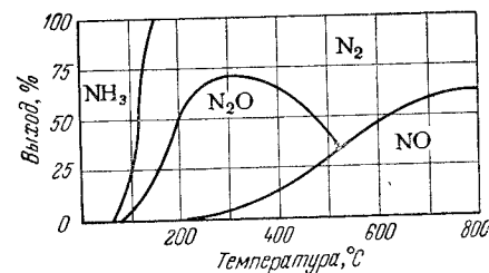
Рис. II-2. Состав газа, образующегося при окислении аммиака на марганцевом катализаторе.
