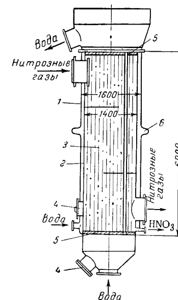
Рис. VI-13. Холодильник-конденсатор: 1 — водяная рубашка; 2 — кожух трубки; 3 — охлаждающие трубки; 4 — лок; 5 — трубные доски; 6 — компенсаторы.
