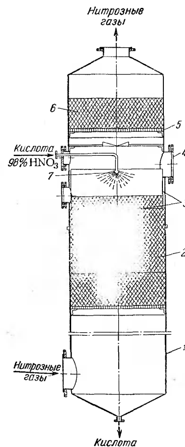
Рис. VIII-28. Доокислитель: 1 — кожух; 2 — насадка; 3 — футеровка (листовой алюминий); 4 — лаз; 5 — решетка; 6 — слой колец для улавливания брызг; 7 — разбрызгиватель.
