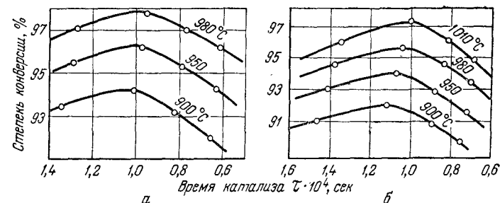
Рис. 11-11. Зависимость степени конверсии NH 3 от времени катализа и температуры: а — давление 10 ат на 20 сетках; б — давление 20 ат на 30 сетках.
