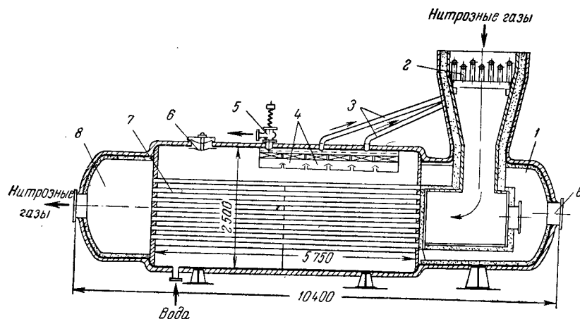
Рис. VI-11. Котел-утилизатор:
