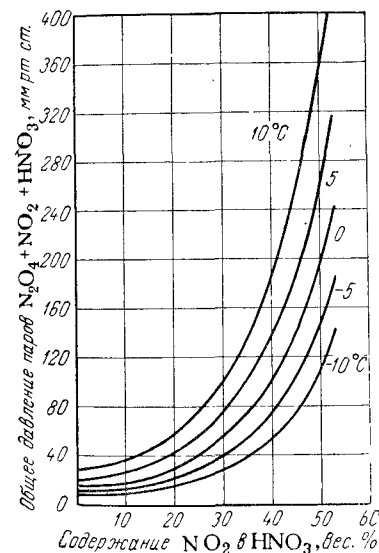
Рис. VIII-3. Общее давление паров N_2O_4 + NO_2 + HNO_3 над раствором четырехоксида азота в 100%-ной HNO_3 .
