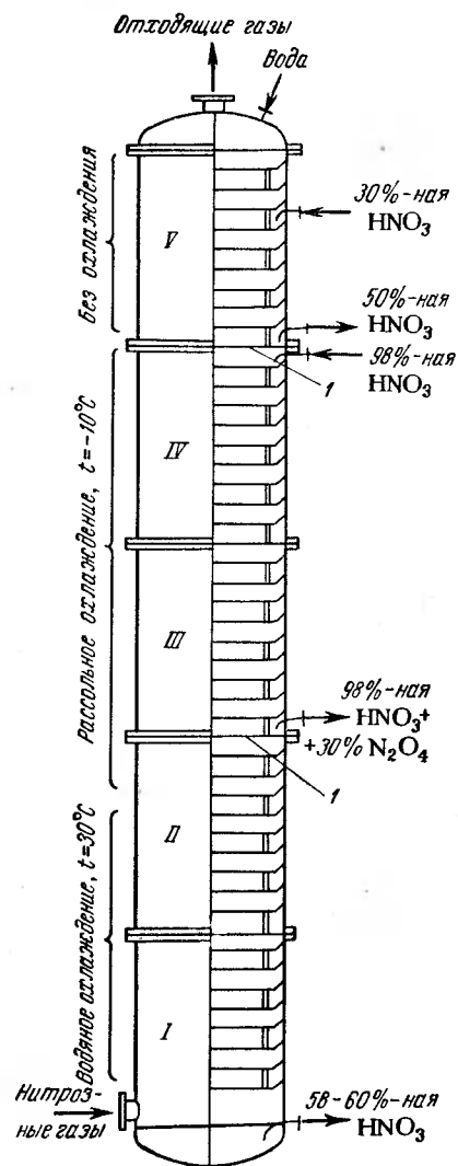
Рис. VIII-41. Схема работы колонны для поглощения окислов азота концентрированной азотной кислотой под давлением от 6 ат и выше:
