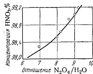
Рис. VIII-23. Зависимость концентрации азотной кислоты от соотношения N_2O_4:H_2O (температура 85—90°С, давление 40 ат).
