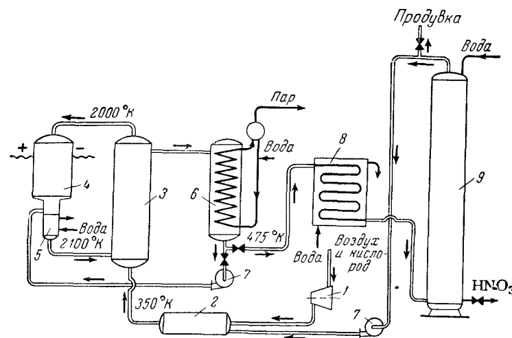
Рис. 1-11. Принципиальная схема получения азотной кислоты из N_2 и O_2 с помощью плазмы под давлением 10 ат:
