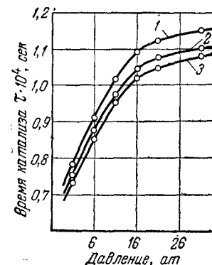
Рис. 11-12. Зависимость времени катализа NH 3 от давления и температуры при максимальном выходе NO: 1 — при 900° С; 2 — при 950° С; 3 — при 980° С.
