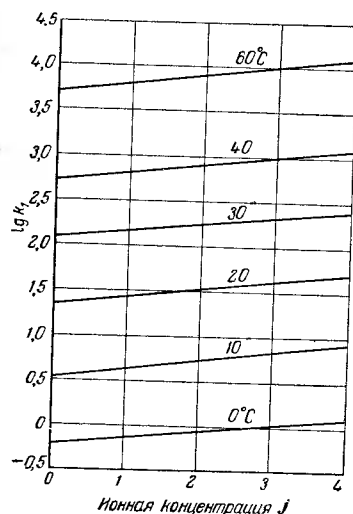
Рис. IV-1. Зависимость константы скорости разложения k_1 азотистой кислоты от температуры и ионной концентрации азотистой кислоты j .
