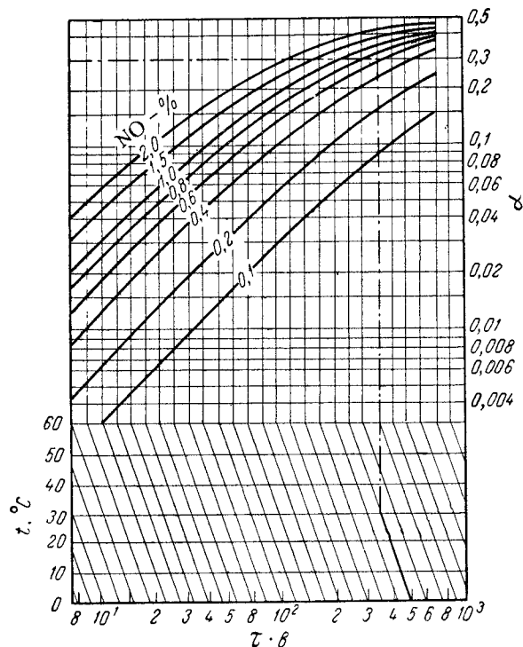
Рис. IX-1. Номограмма для определения степени окисления NO (составлена Л. Мучкай):
