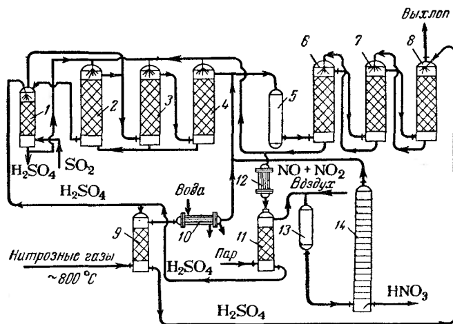
Рис. VII-25. Схема совместного получения серной и азотной кислот по методу В. И. Атрощенко, А. Н. Цейтлина и А. Я. Крайней:
