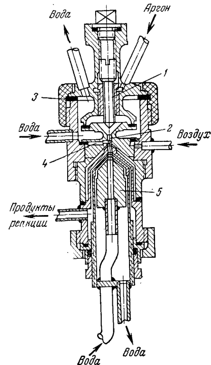
Рис. 1-7. Схема плазмотрона мощностью 45 квт:
