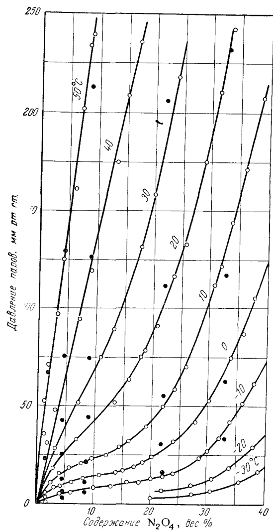
Рис. IV-22. Общее давление паров \text{NO}_2 и \text{N}_2\text{O}_4 над растворами в системе \text{N}_2\text{O}_4 - \text{HNO}_3 при различной температуре.
