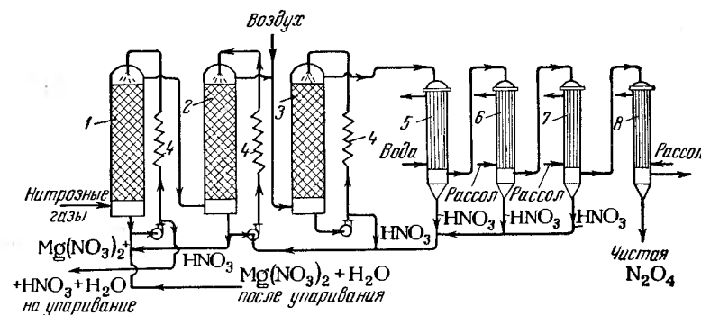
Рис. VIII-42. Принципиальная схема получения чистой четырехокси азота:
