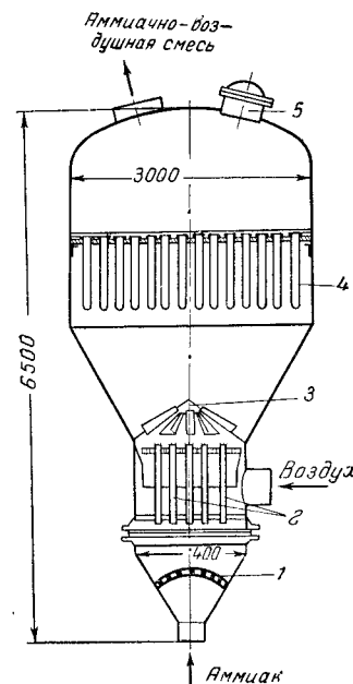
Рис. VI-9. Смеситель и поролитовый фильтр: 1 — распределительная решетка; 2 — трубки для распределения аммиака; 3 — конус-завихритель; 4 — поролитовые трубки.
