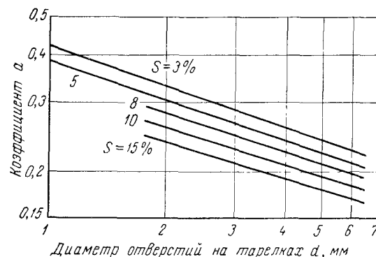
Рис. IV-9. Зависимость коэффициентов \alpha от диаметра отверстий d и доли площади ( S ) сечения этих отверстий от общей площади тарелки.
