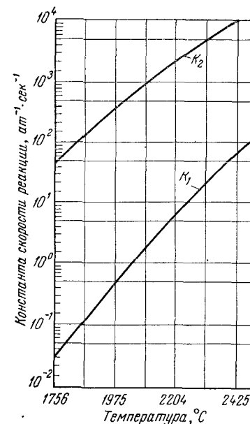
Рис. I-2. Значения констант скоростей k_1 и k_2 .
