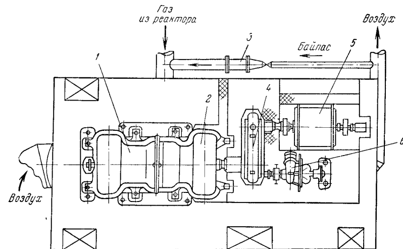
Рис. VI-15. Аппарат ГТТ-3:
