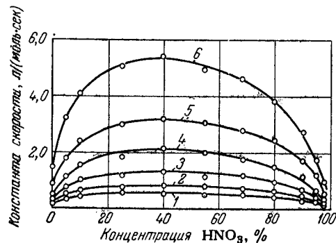
Рис. IV-3. Зависимость константы скорости реакции окисления окиси азота кислородом в водном растворе от температуры (насыщенные растворы получены при 20—25 атм):
