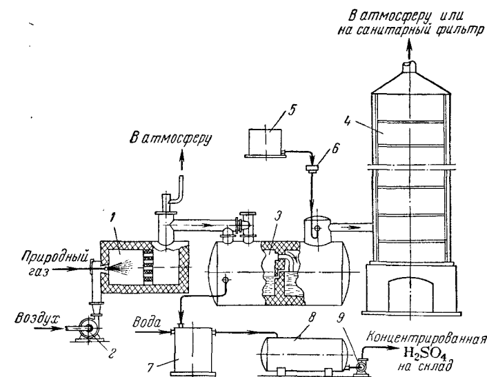
Рис. VII-17. Схема установки концентрирования серной кислоты: 1 — топка; 2 — воздуходувка; 3 — концентратор; 4 — электрофильтр; 5 — напорный бак отработанной серной кислоты; 6 — регуляторная коробка; 7 — холодильник концентрированной H_2SO_4 ; 8 — сборник кислоты; 9 — насос.
