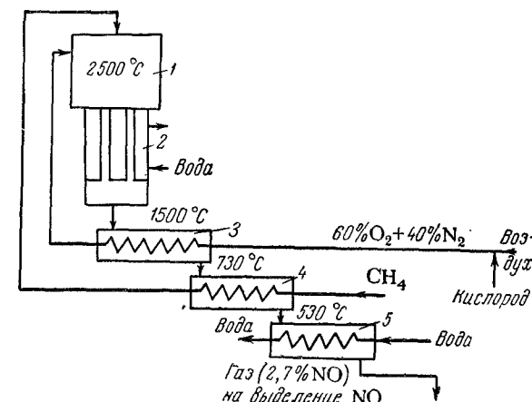
Рис. 1-5. Схема установки синтеза окиси азота путем сжигания метана в воздухе, обогащенном кислородом: 1 — реактор; 2 — холодильник; 3, 4, 5 — теплообменники для использования тепла газов.
