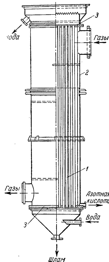
Рис. VI-5. Газовый холодильник: 1 — трубки; 2 — корпус; 3 — трубные решетки.
